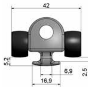
Body 19 mm 1530-19-XX
