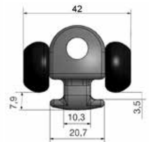
Body 23 mm met grote wiel 1531-23-XX
