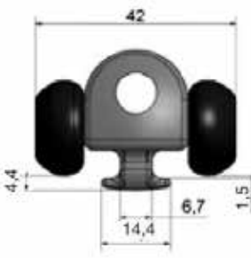
Body 16 mm met grote wiel 1531-16-XX
