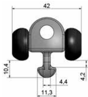
Body 11 mm met grote wiel 1531-11-XX
