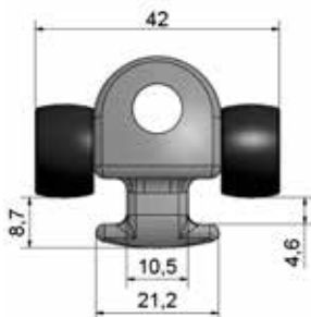
Body 23 mm 1530-23-XX & 1535-23-XX
