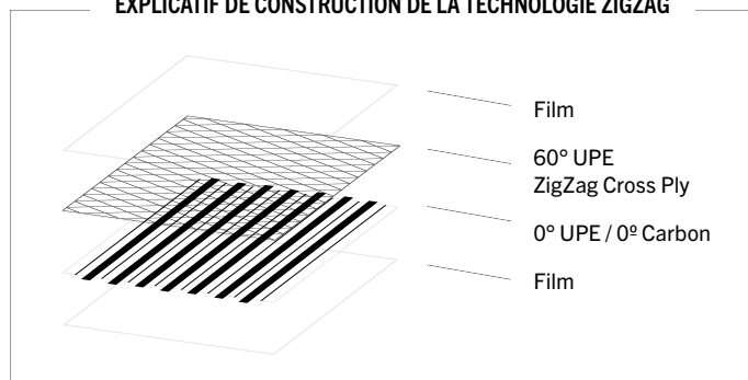
EXPLICATIF DE CONSTRUCTION DE LA TECHNOLOGIE ZIGZAG
